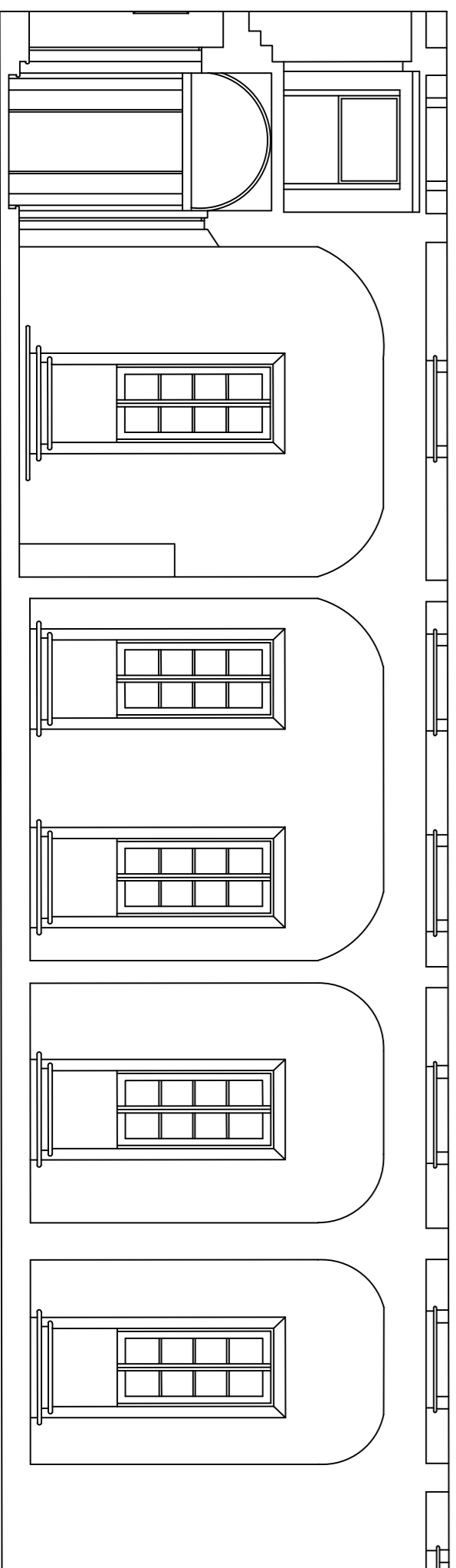
SEZIONE G-G'
